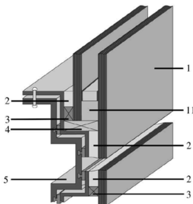
Figura 5: Disegno con vetro isolante sfalsato.
