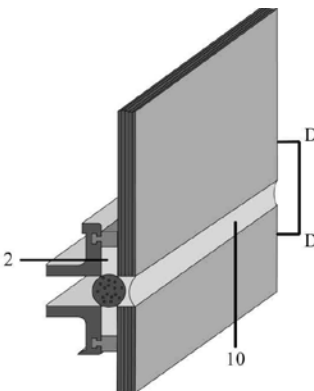
Figura 5: Disegno con vetro isolante sfalsato.
