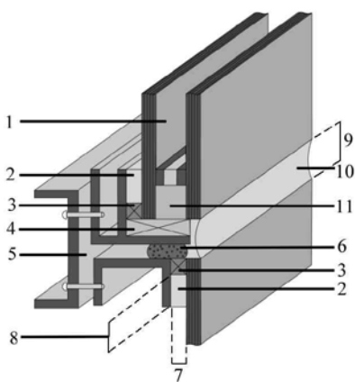
Figura 4: Disegno con vetro isolante supportato.
