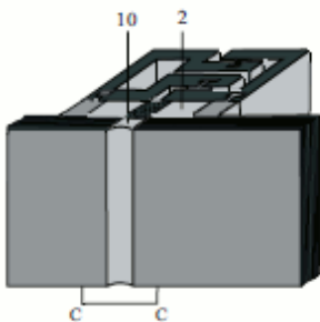
Figura 1B: Sezione DD: disegno a 4 lati - vetro non supportato
