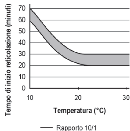
Figura 4: Sigillante DOWSIL 993 - Intervallo tempi di inizio reticolazione
