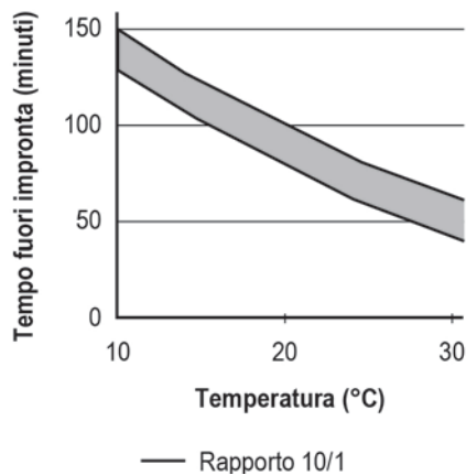
Figura 3: Sigillante DOWSIL 993 - Intervallo tempi fuori impronta
