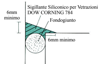
Figura 2: Giunto concavo.
