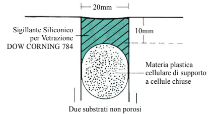
Figura 1: Giunto profondo.
